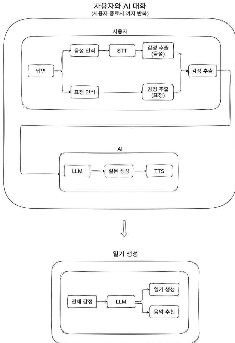
그림2. 시스템 흐름 다이어그램
