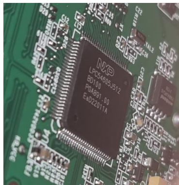
[그림 3-9. Corsair K70 RGB TKL의 MCU]
